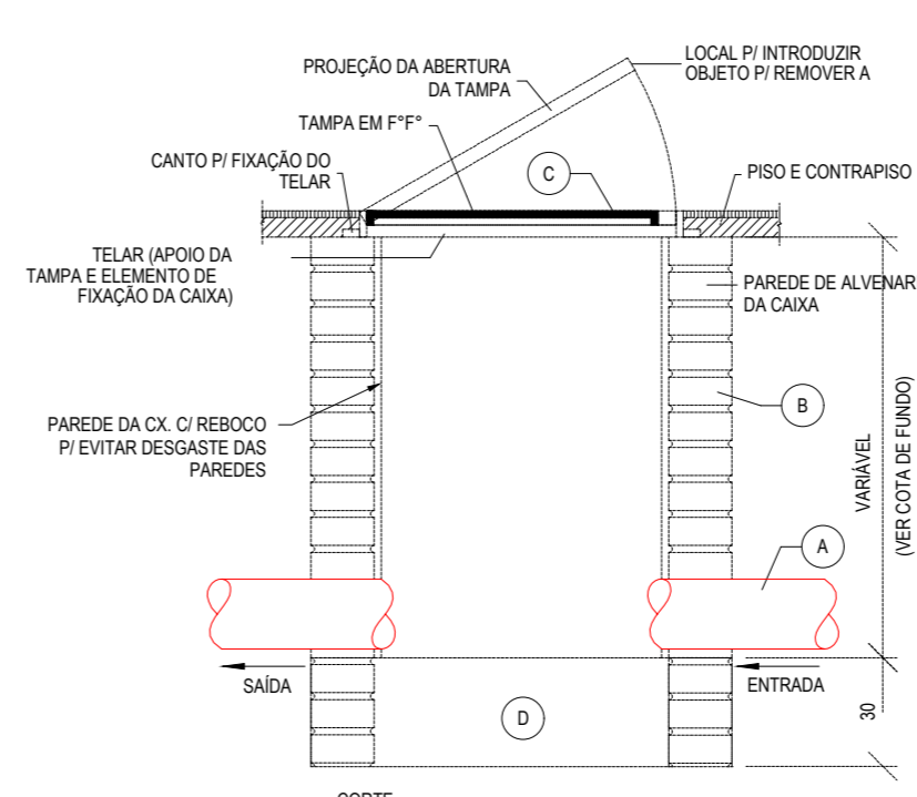
DETALHE CAIXA PASSAGEM SEM ESCALA
