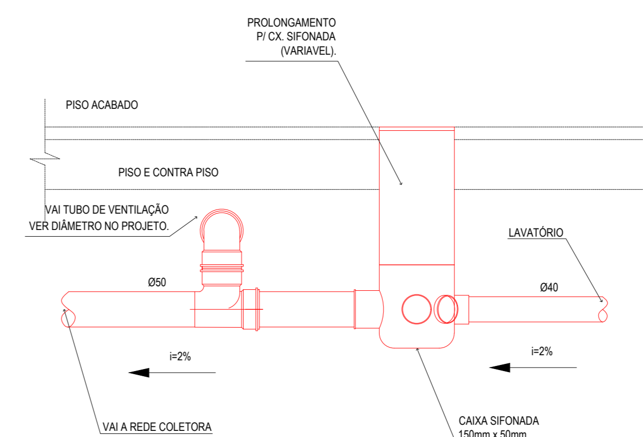
DETALHE CAIXA SIFONADA SEM ESCALA
