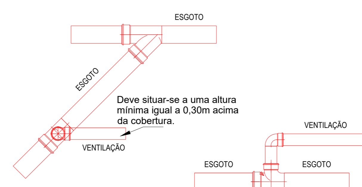
DETALHE TUBO DE VENTILAÇÃO SEM ESCALA
