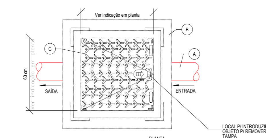
DETALHE CAIXA SIFONADA SEM ESCALA
